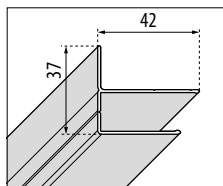
WALL 2P - G - B - S2 - 3P - 2A
