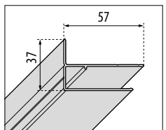
EXTENSION 2P - G - B - S2 - 3P - 2A
